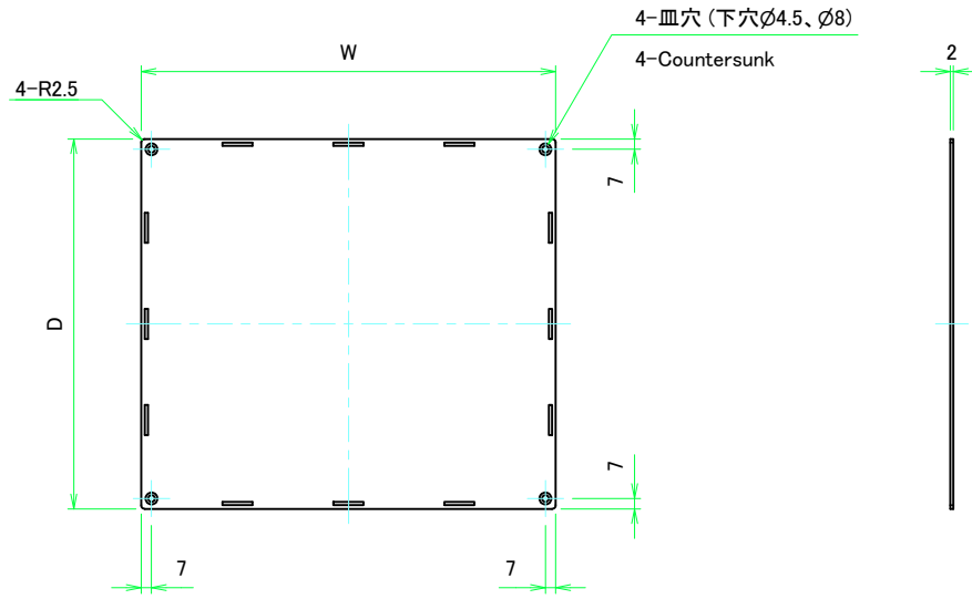
上カバー表面 / Top cover Frontside
