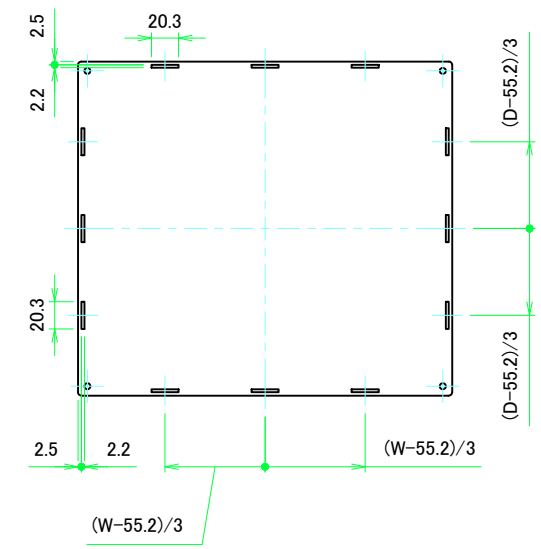
上カバー裏面 / Top cover Backside
